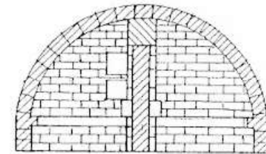
Coupe D-D
