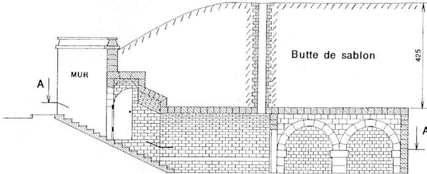
Vue de profil selon coupe B-B
