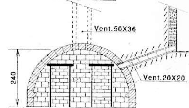
Coupe D-D
